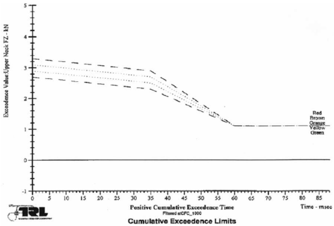
[Fig. 3-1: Tensile Load]
