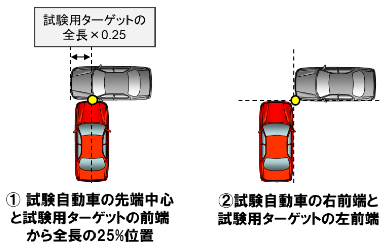
図5 交差点条件
