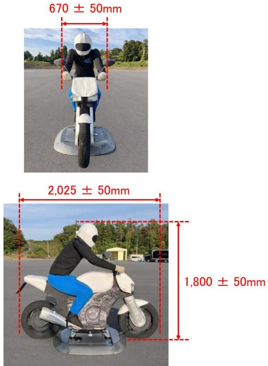
付図 A 試験用ターゲットの外観と寸法諸元
