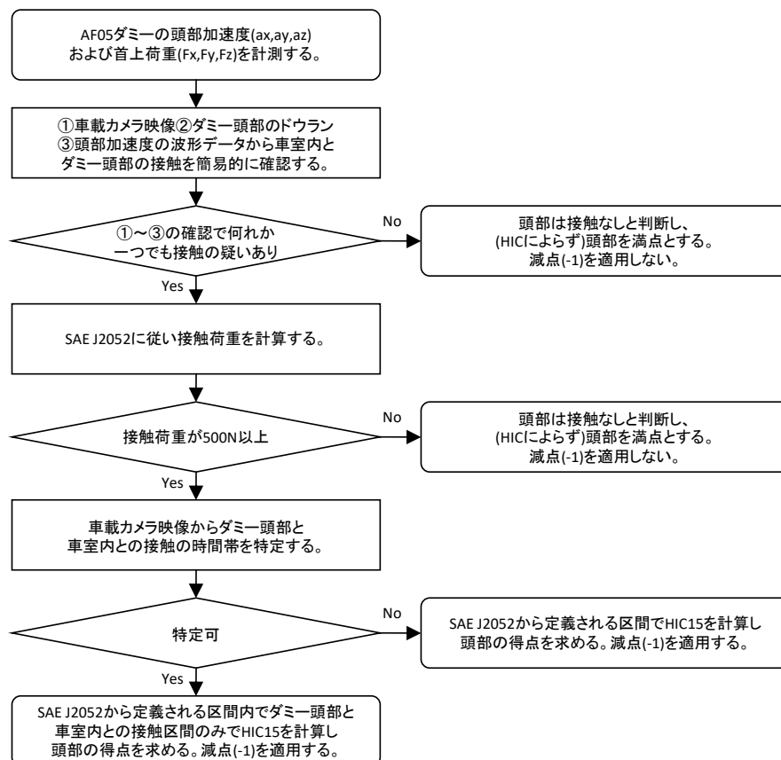
図3 頭部二次衝突判定フローチャート
