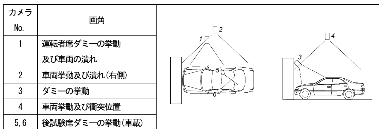
図 7 高速度カメラの撮影範囲
