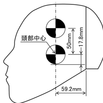
図2 ダミー頭部のターゲットマーク貼付例
