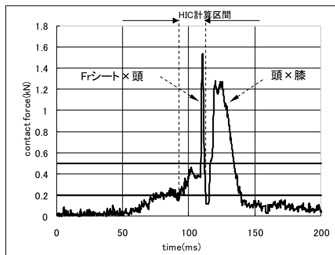
図4 接触荷重を分離でき、HIC 計算区間も分離可能な例
