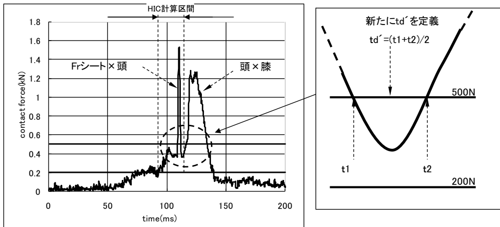
図5 接触荷重は分離できるが、HIC 計算区間の分離が不可能な例
