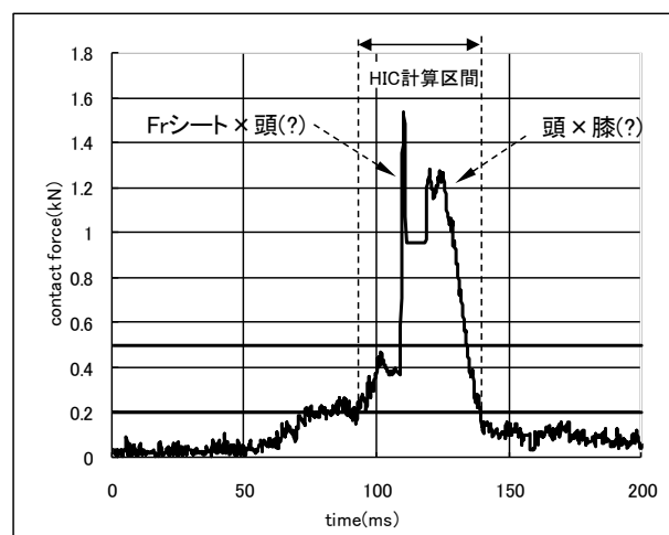
図6 接触荷重の分離が出来ない例
