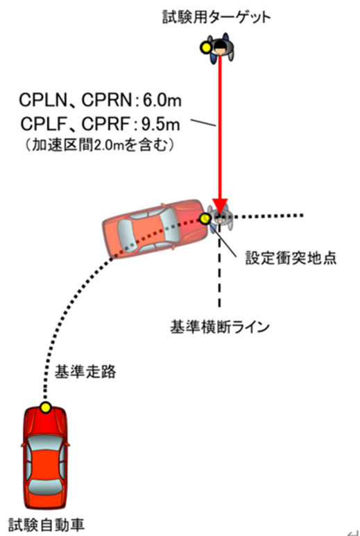
図 4 試験用ターゲットの初期位置
