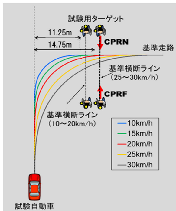
図 3-2 CPRN 及び CPRF シナリオ
