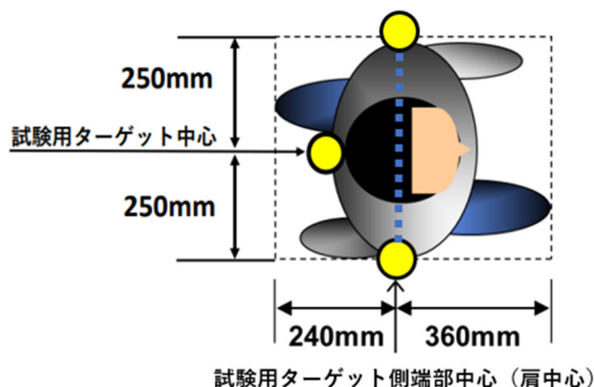
図 1 試験用ターゲット中心の定義
