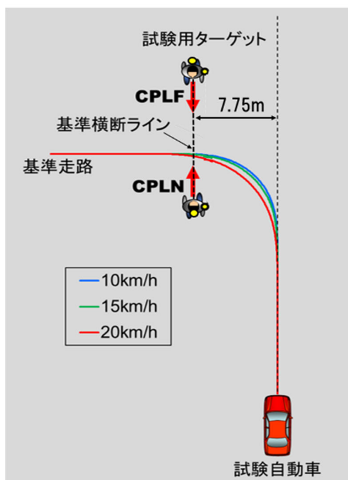
図 3-1 CPLF 及び CPLN シナリオ
