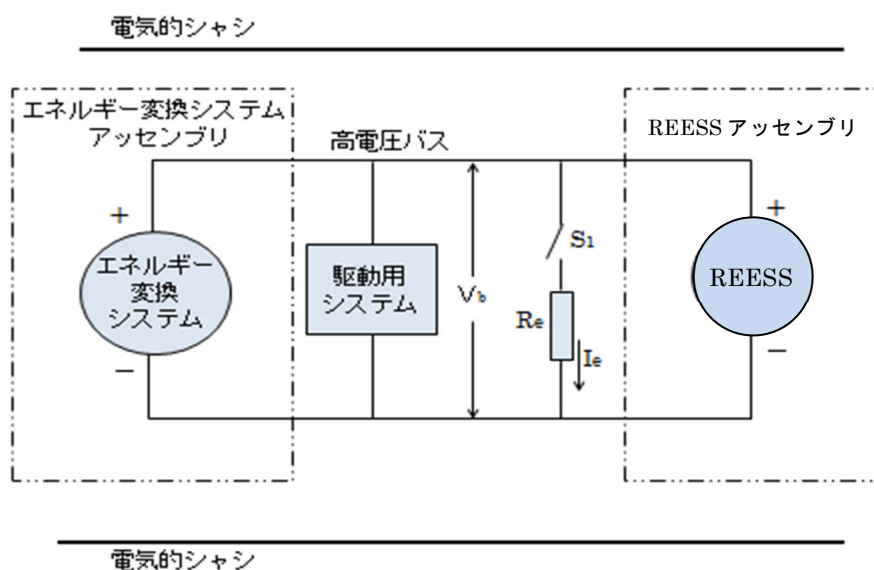
図 1（例：X コンデンサに貯蔵された高電圧バスエネルギーの測定）
