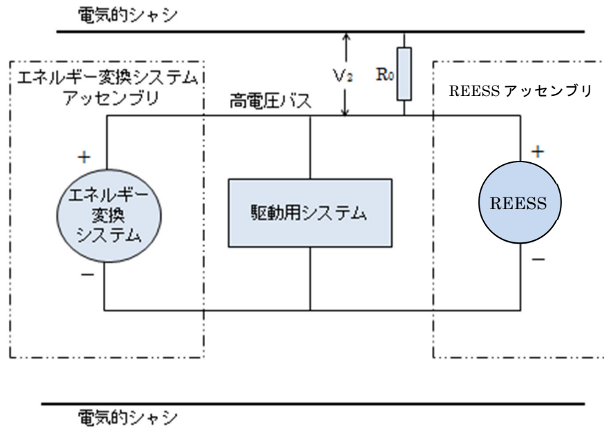
図 2 ( V_2' の測定)
