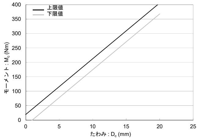
(a) 大腿骨曲げ変形コリドー
