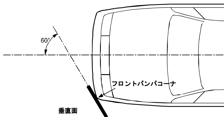
図 3.1 フロントバンパコーナ
