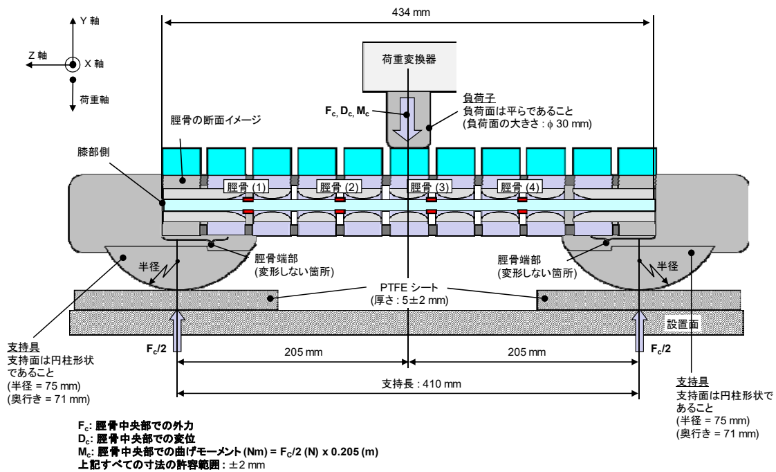
図8 大腿骨の静的検定試験セットアップ
