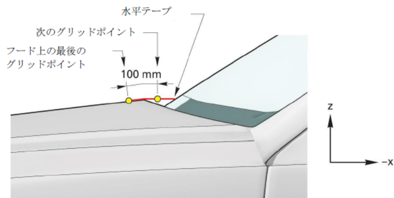
図 3.10 外部輪郭の下グリッドポイント (車両中心線上までの例)
