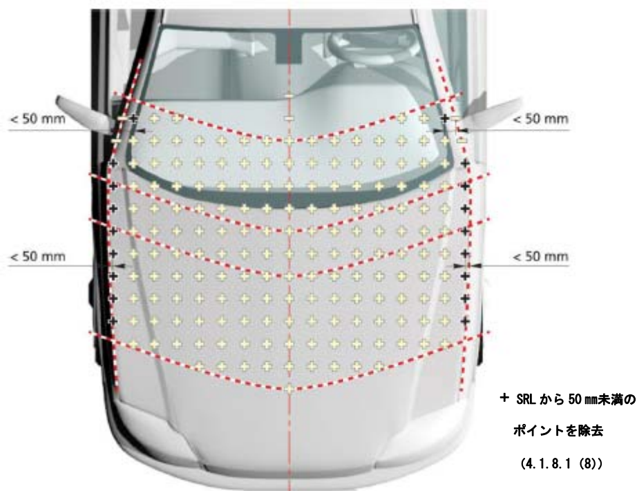
図 3.11 グリッドポイントの削除
