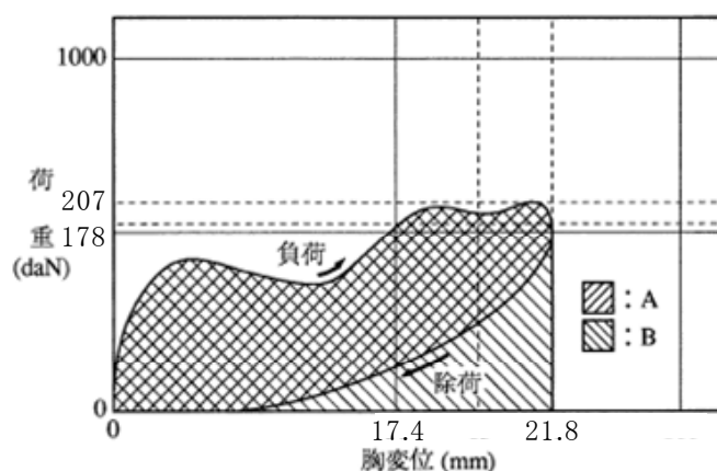
図9 胸部特性試験荷重－変位曲線
