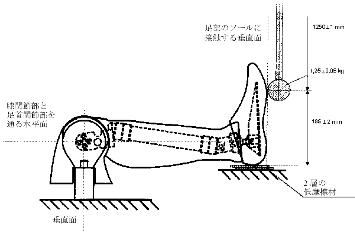
図 11 下足部衝撃試験（靴なし）（試験装置仕様）
