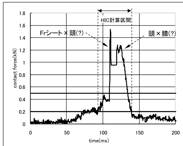
図7 接触荷重の分離が出来ない例
