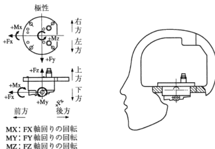
図11 6軸型首部荷重計取付状況
