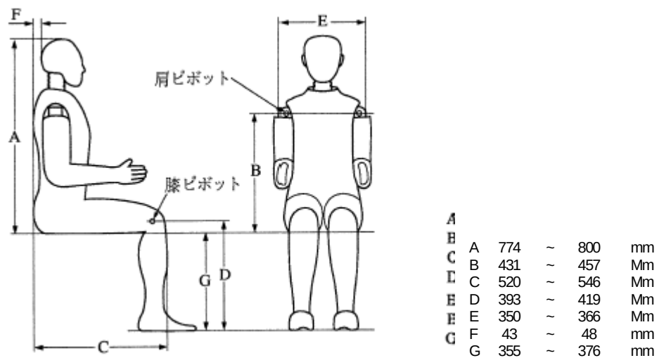
図1 ハイブリッドⅢ構造寸法
