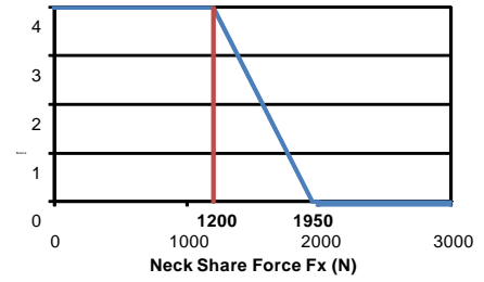
【図 11-2 : 剪断荷重】
