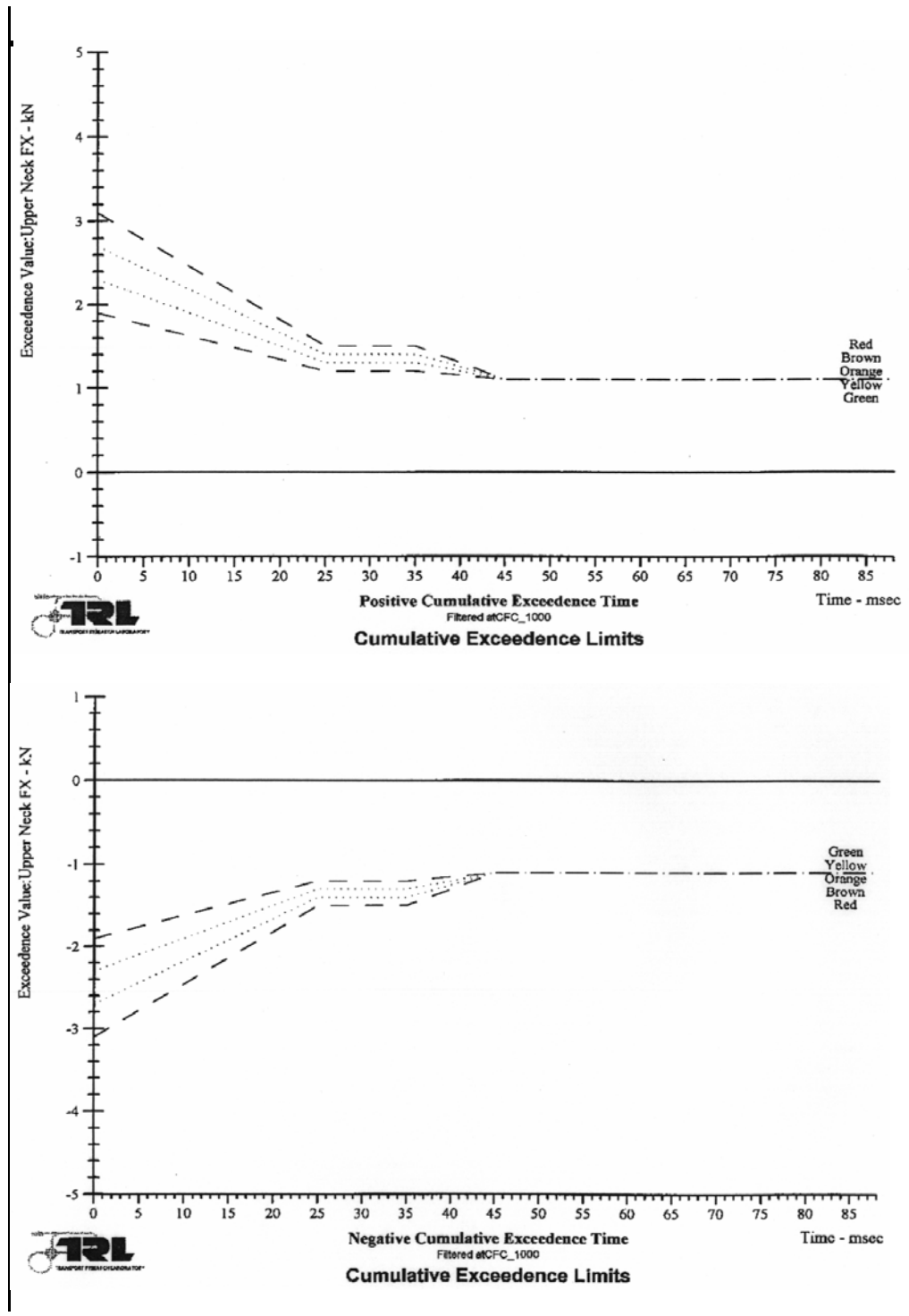
【图 3-2-1：剪断荷重（1）（上図）】 【图 3-2-1：剪断荷重（2）（下図）】
