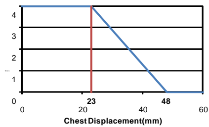
【図 12-2 : 胸部変位量】
