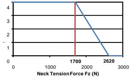
【図 11-1 : 引張荷重】
