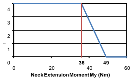
【図 11-3 : 伸張モーメント】
