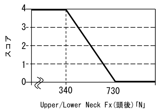
【図 20： 頸部剪断荷重：前後】
