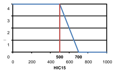
【図 10：頭部傷害値】
