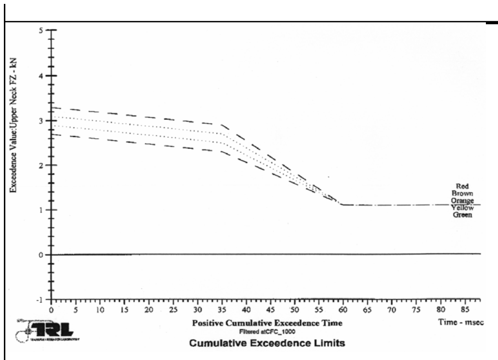
【図 3-1：引張荷重】
