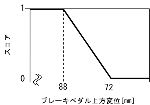
【図 8：ブレーキペダル上方移動量】
