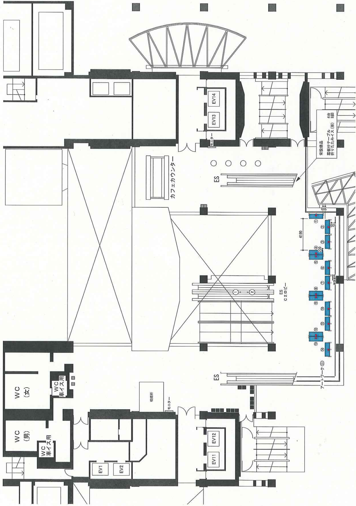
C2ロビー 全体平面図 縮尺 1/200 (A3size)
